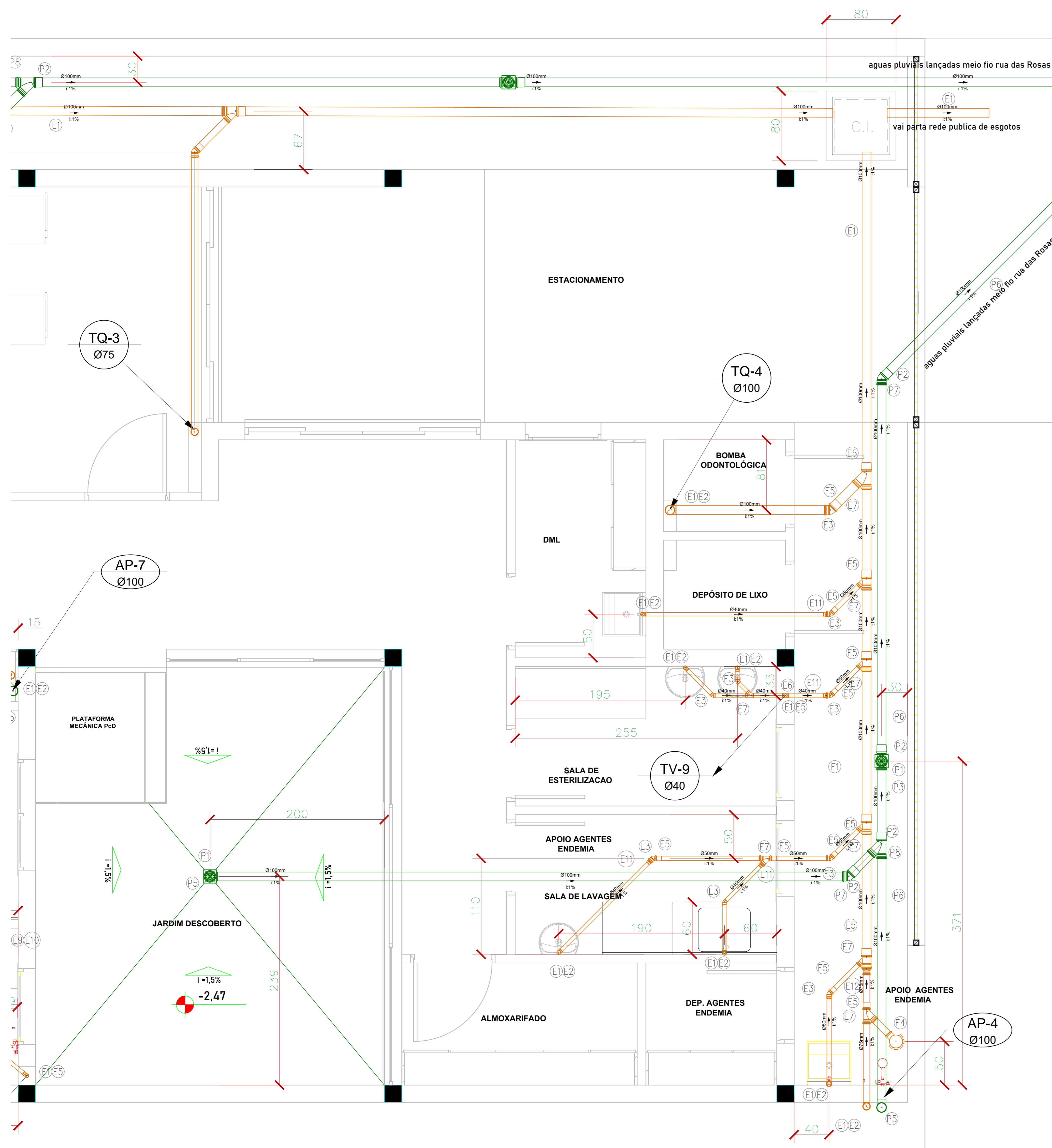
1 DETALHE ESGOTO ÁGUAS PLUVIAIS PAVIMENTO INFERIOR escala 1/25
